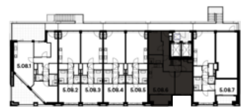
8 E VERDIEPING
