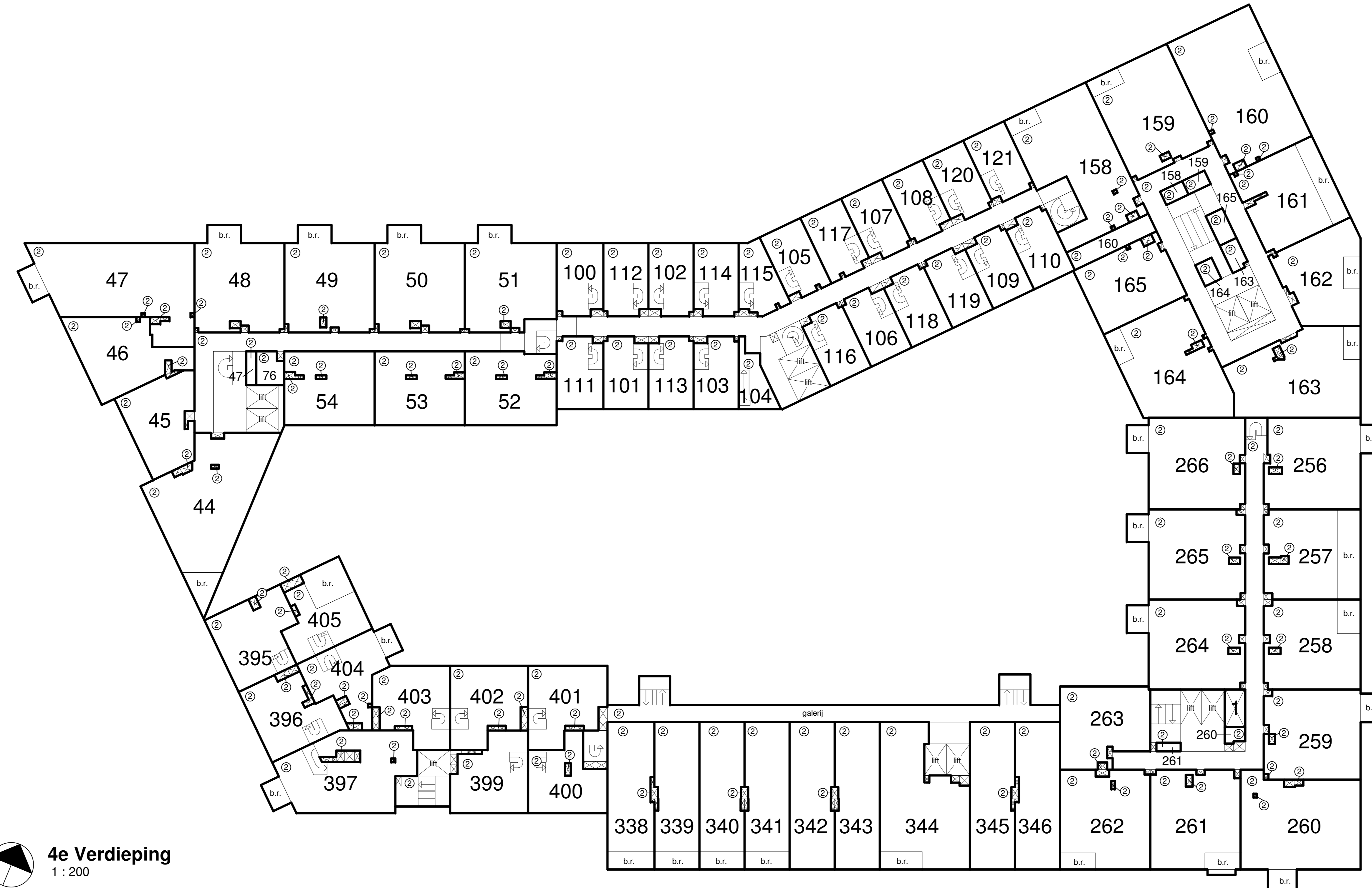
3e Verdieping 1 : 200
