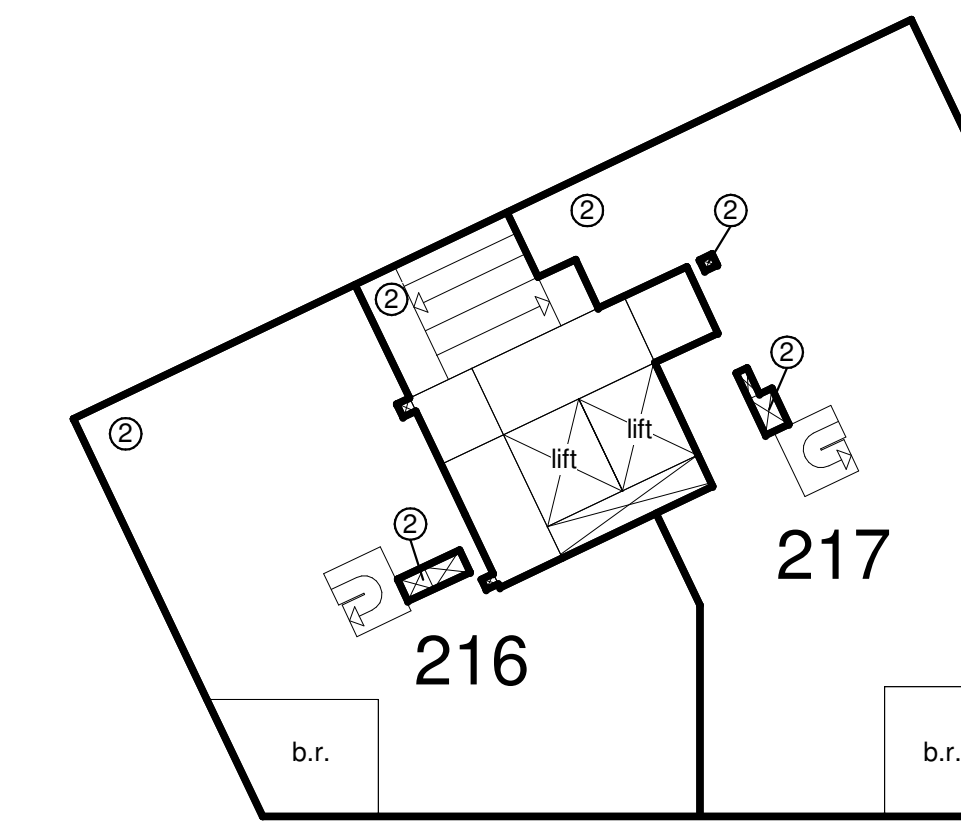
13e Verdieping 1 : 200
