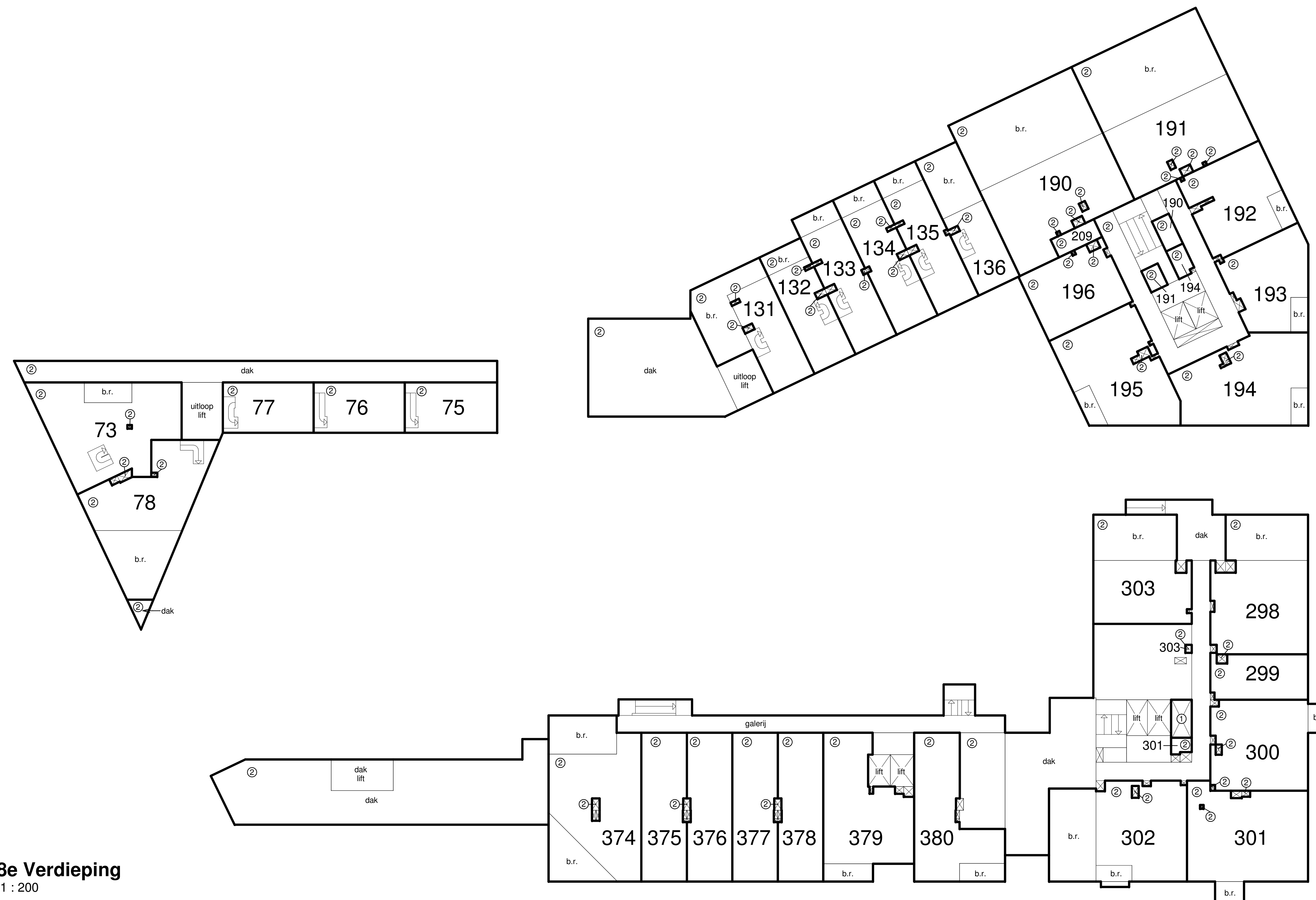
7e Verdieping 1 : 200
